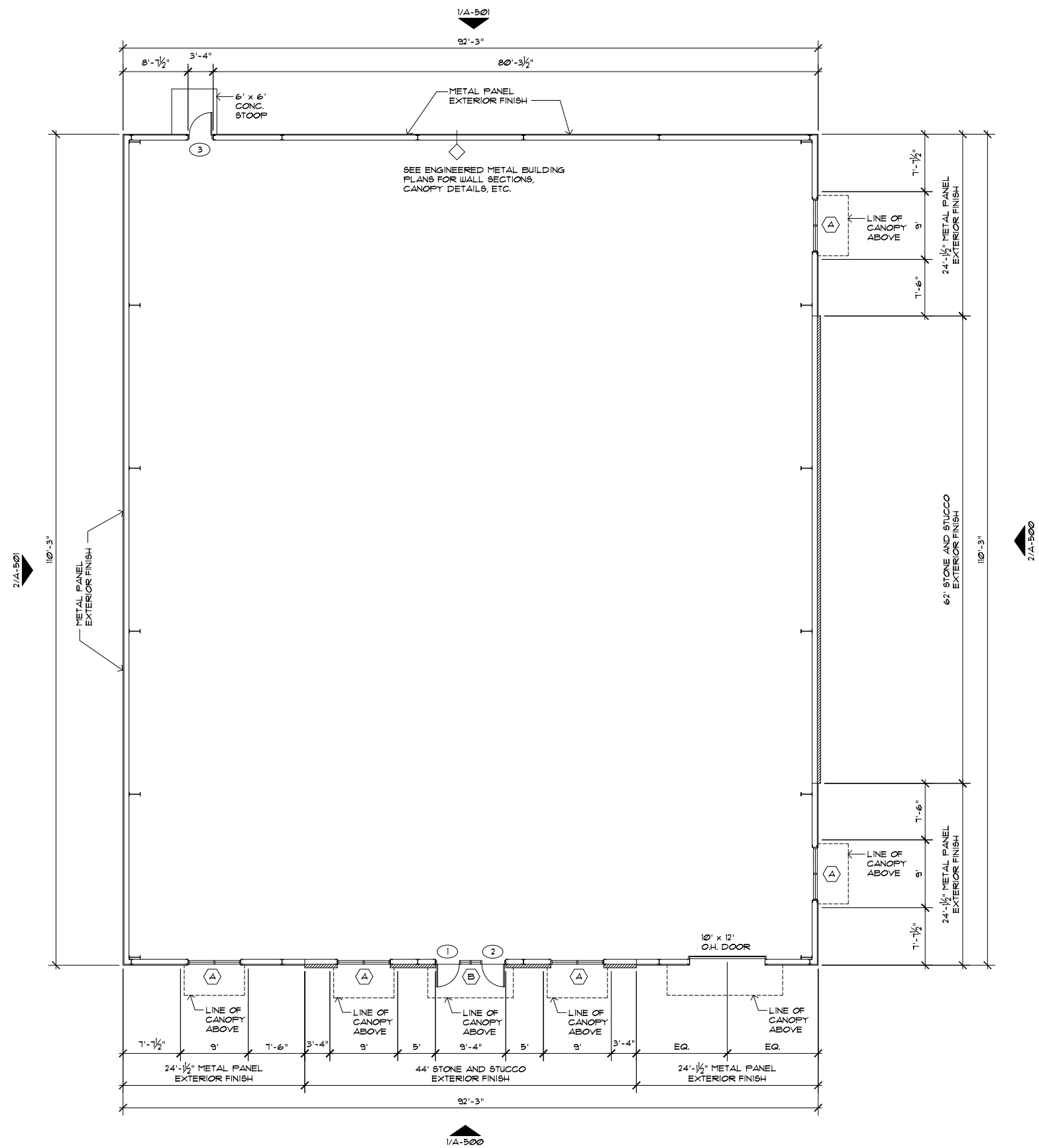
1 FLOOR PLAN SCALE: 1/8" = 1'-0"
